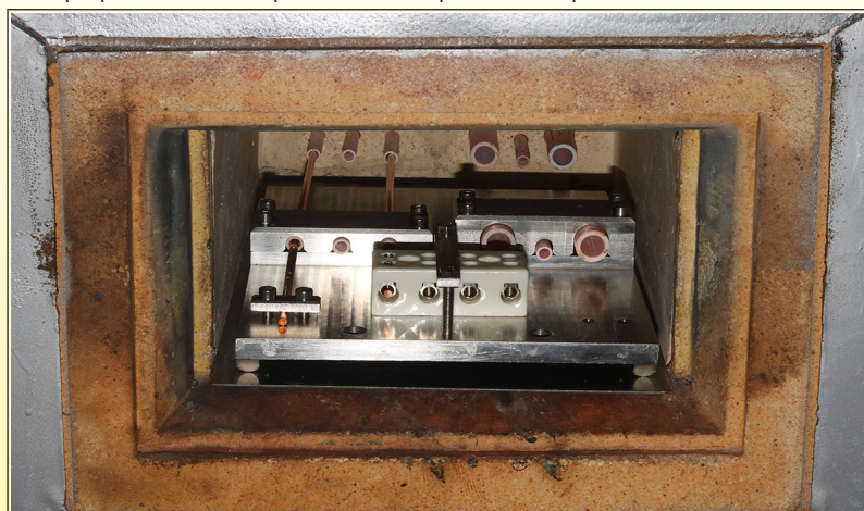
Four d'essai de la résistivité des céramiques en fonction de la température (Laboratoire Ultimheat)
