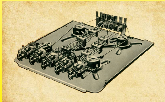
Cablage électrique de la partie supérieure d'une cuisinière électrique Arthur Martin (Catalogue 1949, Musée Ultimheat). Les pièces isolantes en stéatite et en porcelaine sont omniprésentes
